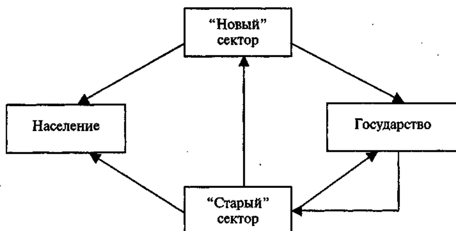
Рис. 4.3. Двухсекторная модель переходной экономики
