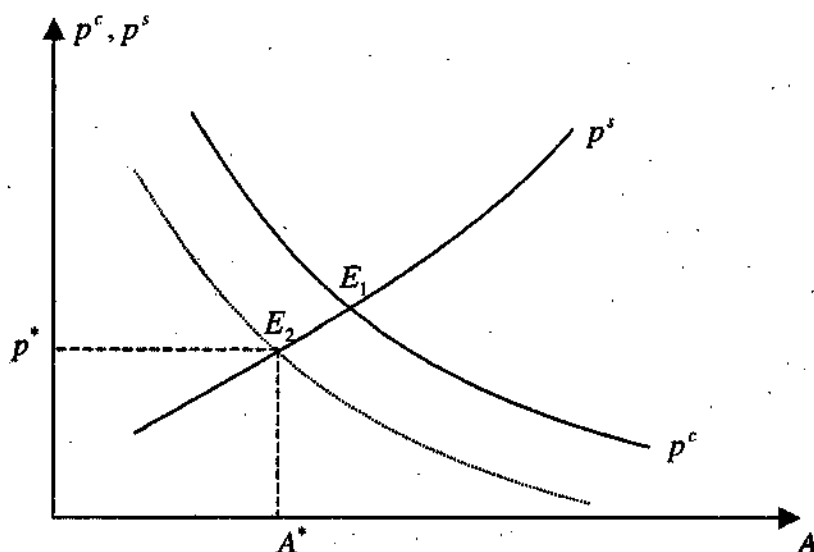
Рис. 2.4. Равновесия в системе моральных рисков
